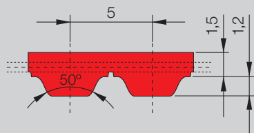
SYNCHROFLEX® зубчатый ремень (SFX) АТ 5 GEN III
