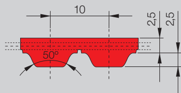
SYNCHROFLEX® зубчатый ремень (SFX) АТ 10 GEN III
