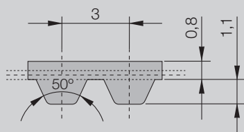
SYNCHROFLEX® зубчатый ремень (SFX) AT 3
