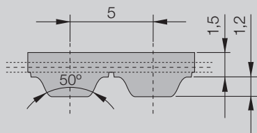
SYNCHROFLEX® зубчатый ремень (SFX) AT 5
